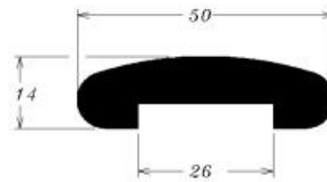
U-430 1.320 kg/m
