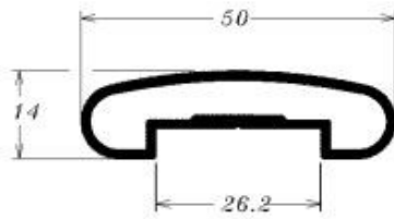
D-095 0.550 kg/m
