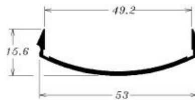
CG-074 0.294 kg/m
