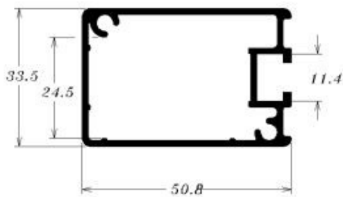
CG-077 0.842 kg/m
