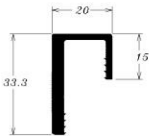
CG-075 0.521 kg/m
